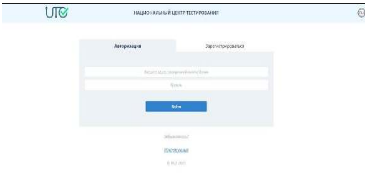
Рисунок 2 - Страница авторизации/регистрации
